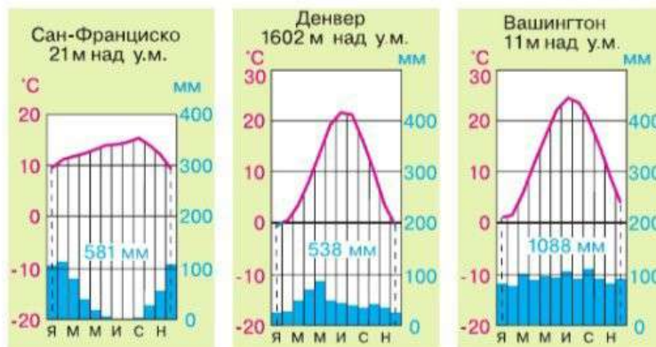
Рис. 153. Климатические диаграммы
