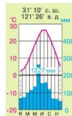
Рис. 194. Климатическая диаграмма
