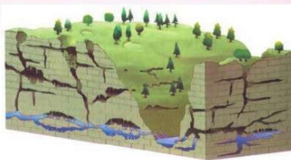
Рис. 160. Карст
