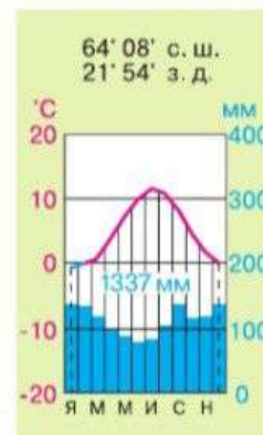
Рис. 171. Климатическая диаграмма
