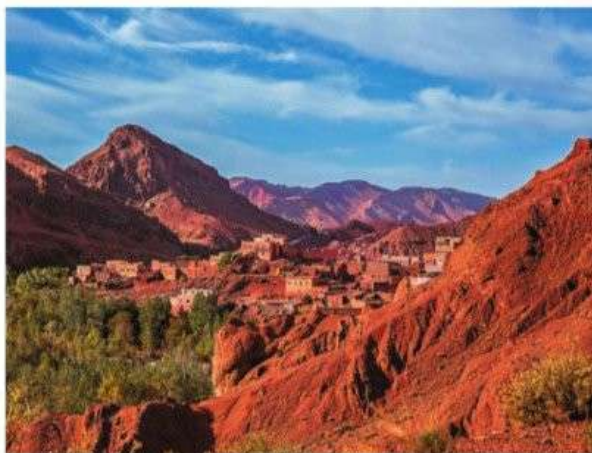
Рис. 76. Атласские горы
