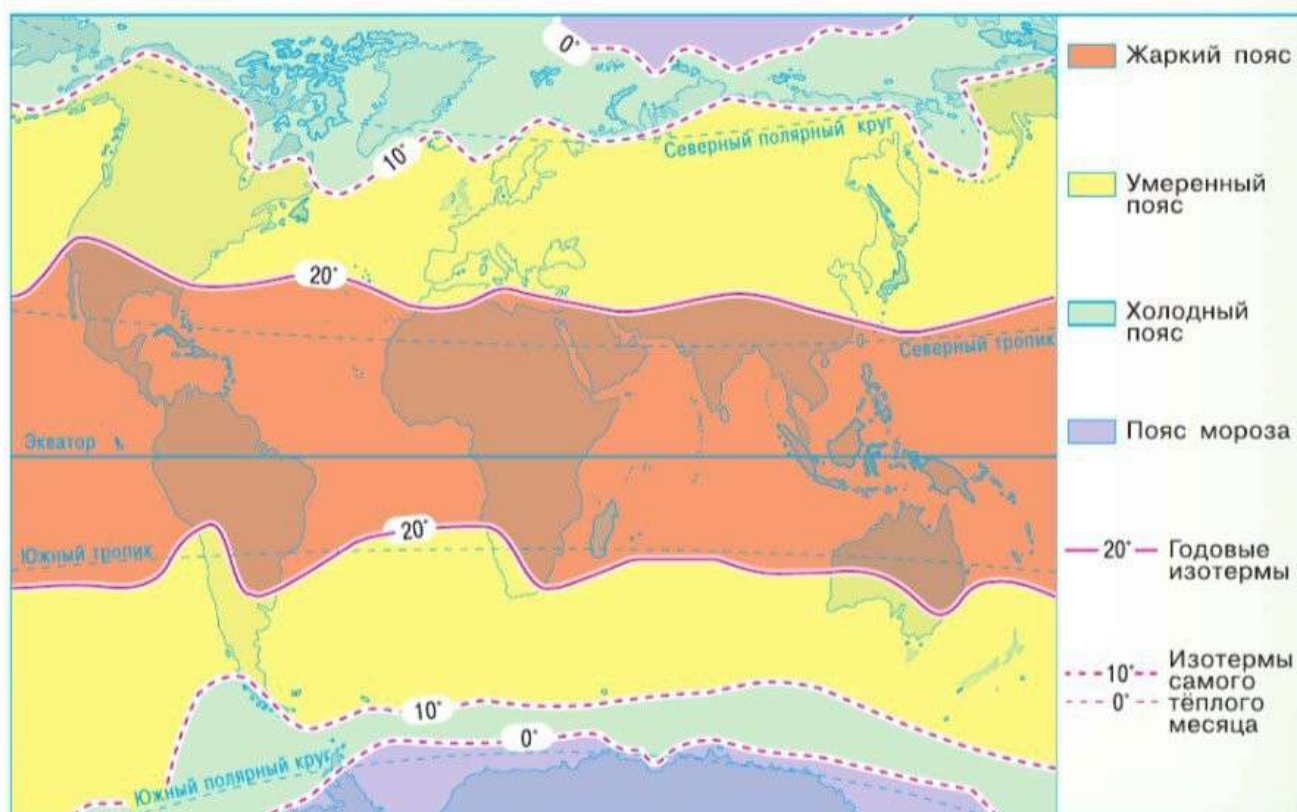
Рис. 27. Тепловые пояса
