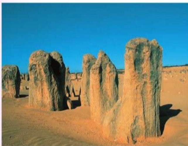
Рис. 96. Австралийская пустыня
