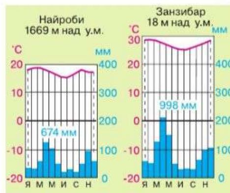
Рис. 84. Климатические диаграммы
