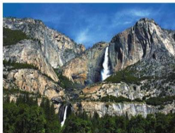
Рис. 137. Водопад Йосемити
